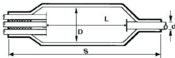
Маркировка муфт и основные размеры в мм
